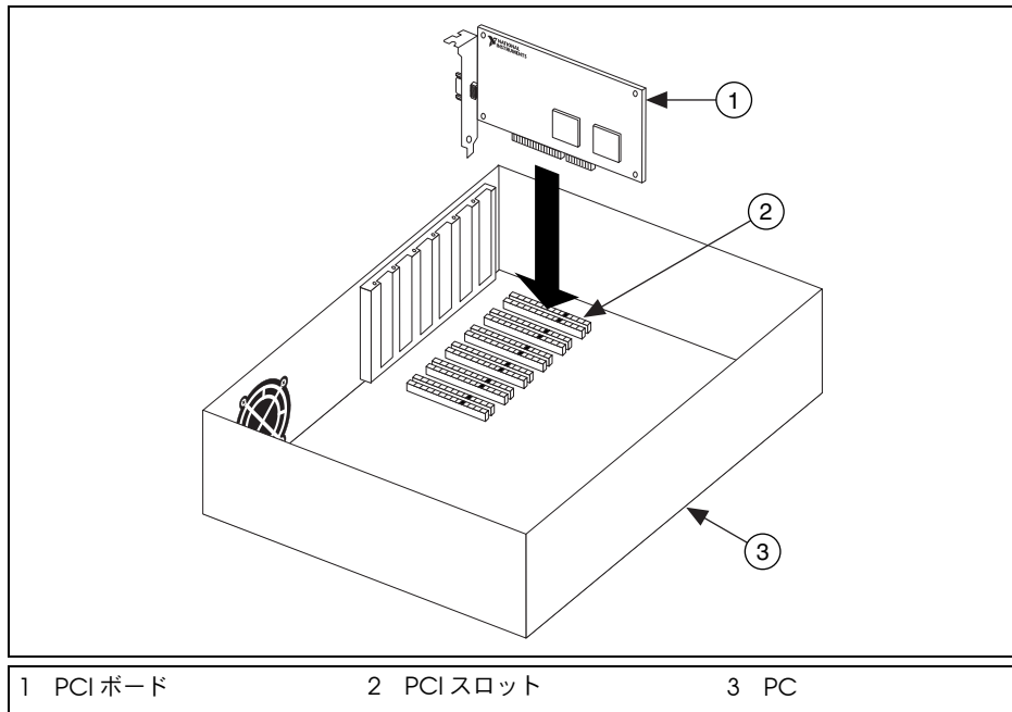
図 16 PCI カードをインストールする
