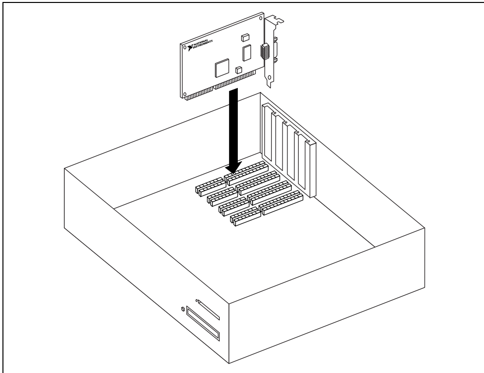
図 13 AT-GPIB/TNT (PnP) または AT-GPIB/TNT+ の取り付け方法
